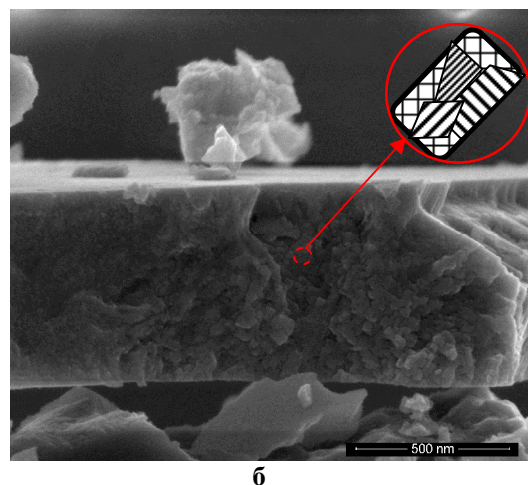
Рис. 1. XRD-спектр зразка \text{WO}_3 (а), після осадженого (1) та після відпалу (2) і SEM зображення плівки після відпалу (б). На вставці схематично зображено зерно з кількома областями когерентного розсіювання X-променів
