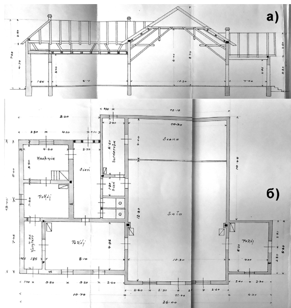
Іл. 7. Розріз (а) та план (б) галицької сокільні, поч. XX ст. ДАІФО. Ф-2. Оп. 8. Спр. 2813. Арк. 1.
