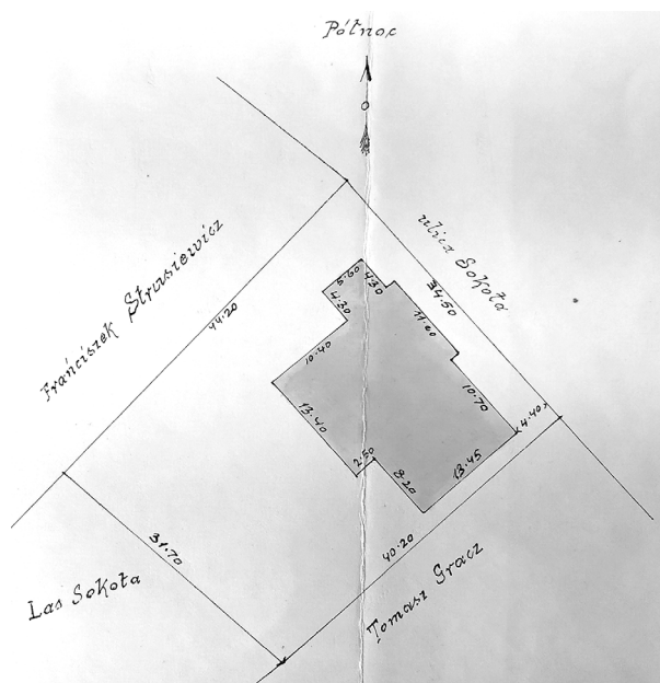
Іл. 3. План-схема території соколиного гнізда у Галичі, поч. XX ст. ДАІФО. Ф-2. Оп. 8. Спр. 2813. Арк. 1.
